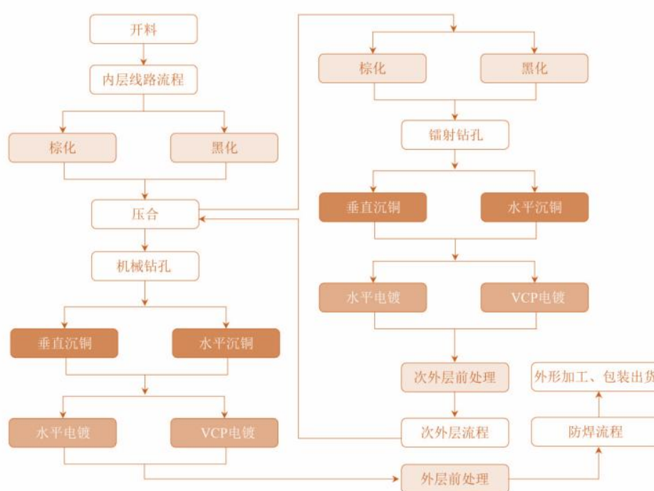
图表 3 减成法和半加成法的主要工艺流程
