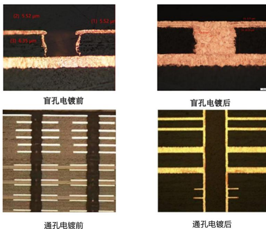
图表 6 电镀效果图
