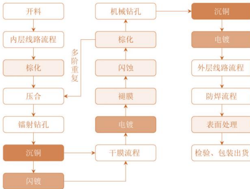
图表 4 PCB 半加成法的主要工艺流程
